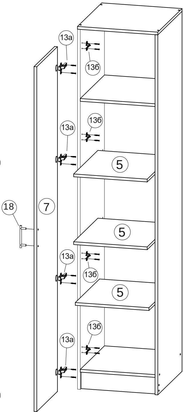
Рис.3 - Монтаж чашки петли 13а на фасад
