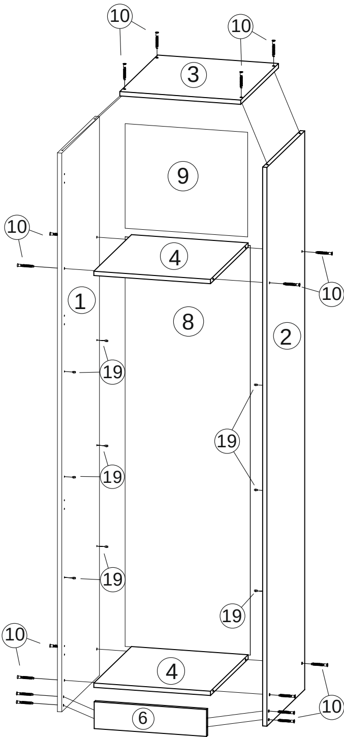
Рис.1 Сборка
