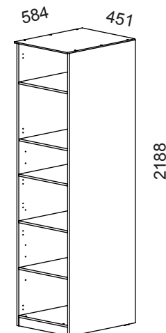
Каркас шкафа для белья ТД 297.07.01 ПМ-297.07.00.000
