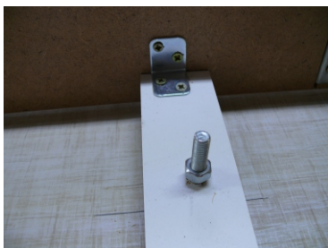
Крепление бруса
