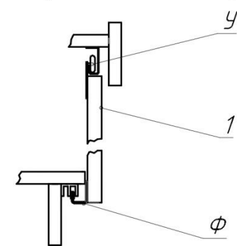
Схема установки дверей
