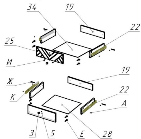
Сборка ящиков
