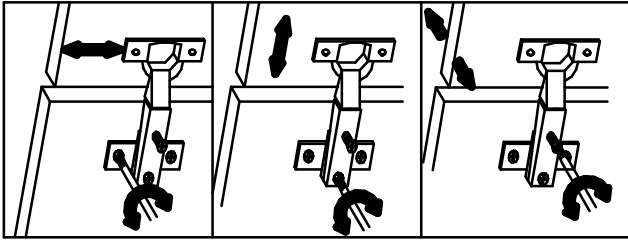
Регулировка дверей
