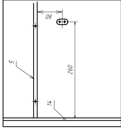
Установка штанги
